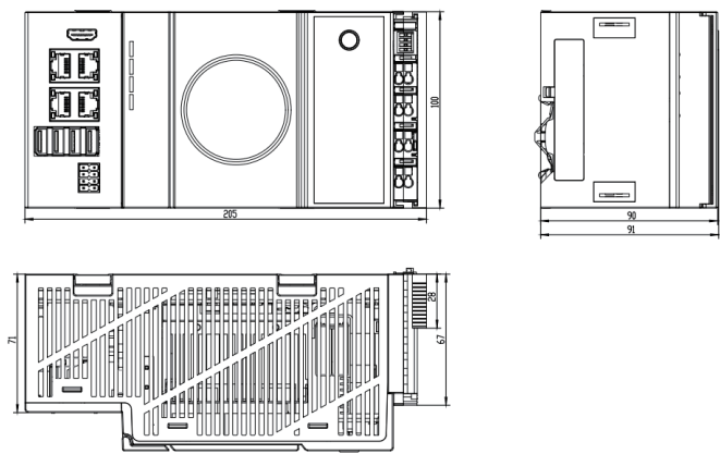
SX21标准型工控机产品尺寸图
