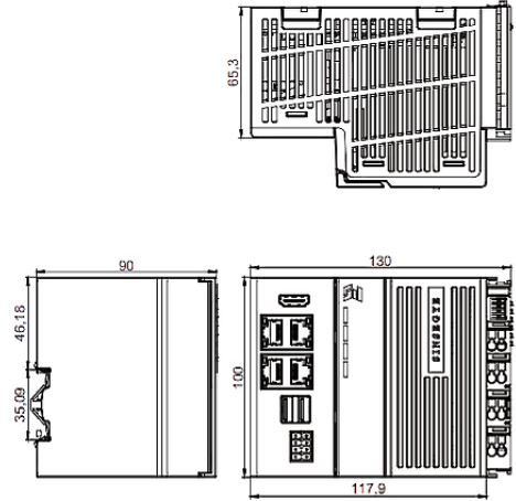
SX51紧凑型工控机产品尺寸图
