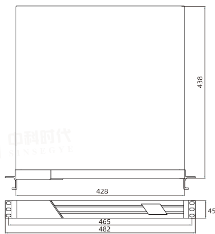
SP5010系列IPC型工控机 产品尺寸图
