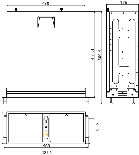
SP5040系列IPC型工控机 产品尺寸图
