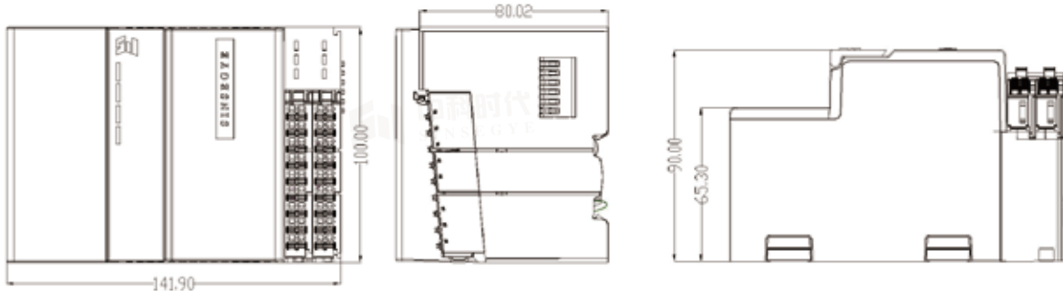
SX52系列紧凑型工控机产品尺寸图
