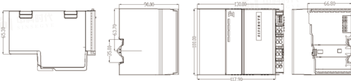
SX51紧凑型工控机产品尺寸图
