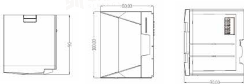
SX58紧凑型工控机产品尺寸图
