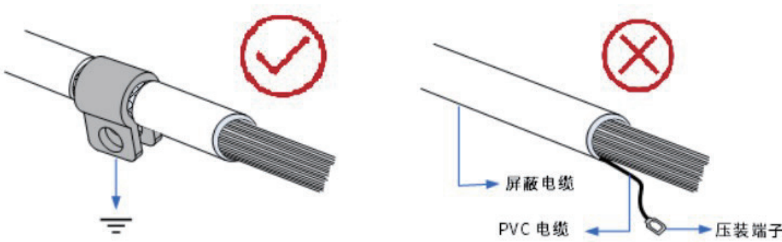
屏蔽线缆接地要求示意图 1
