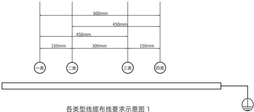
各类型线缆布线要求示意图 1
