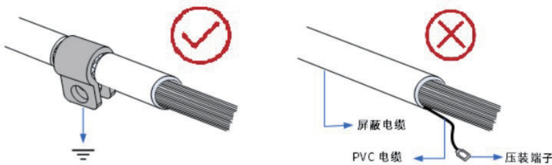
屏蔽线缆接地要求示意图 1
