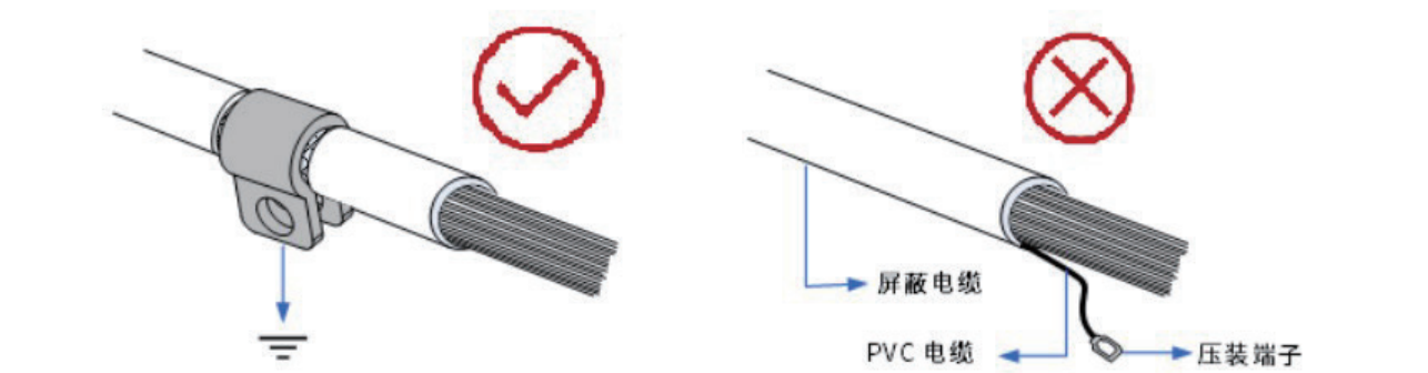
屏蔽线缆接地要求示意图 1
