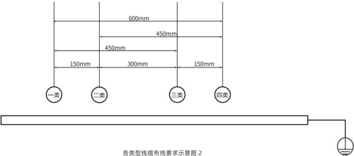
各类型线缆布线要求示意图 2
