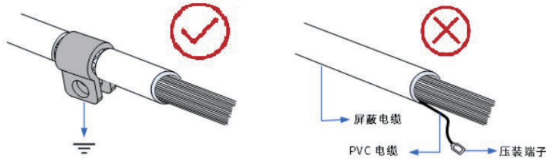
屏蔽线缆接地要求示意图 1
