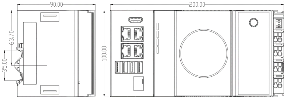
SX21系列产品尺寸图
