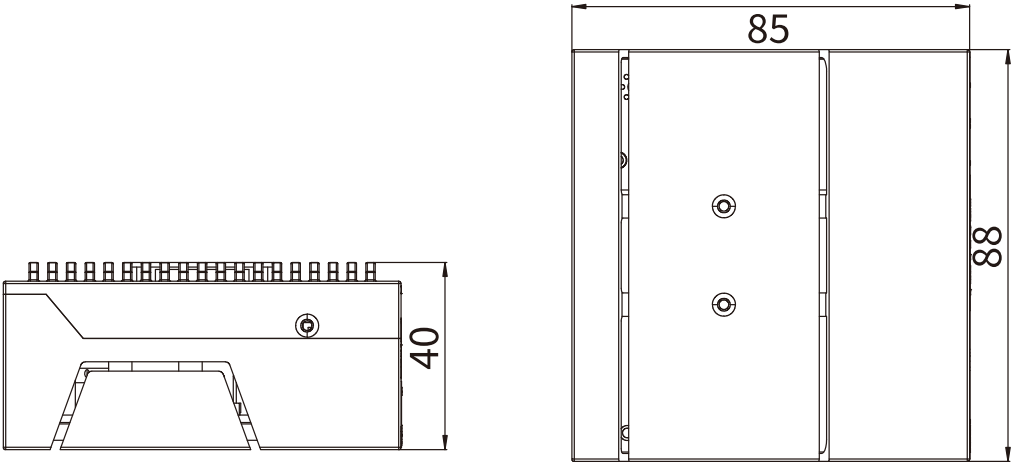
SP6000 安装尺寸（单位：mm）
