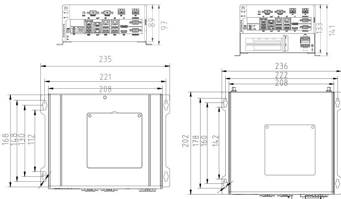
SP7020系列安装尺寸（单位：mm）
