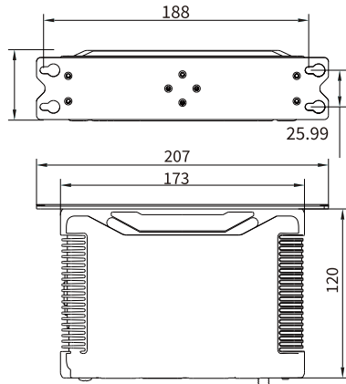
SP7010系列安装尺寸（单位：mm）
