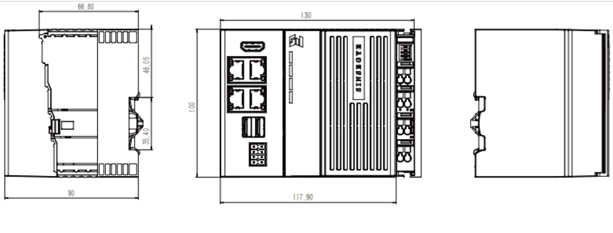
SX51系列产品尺寸图
